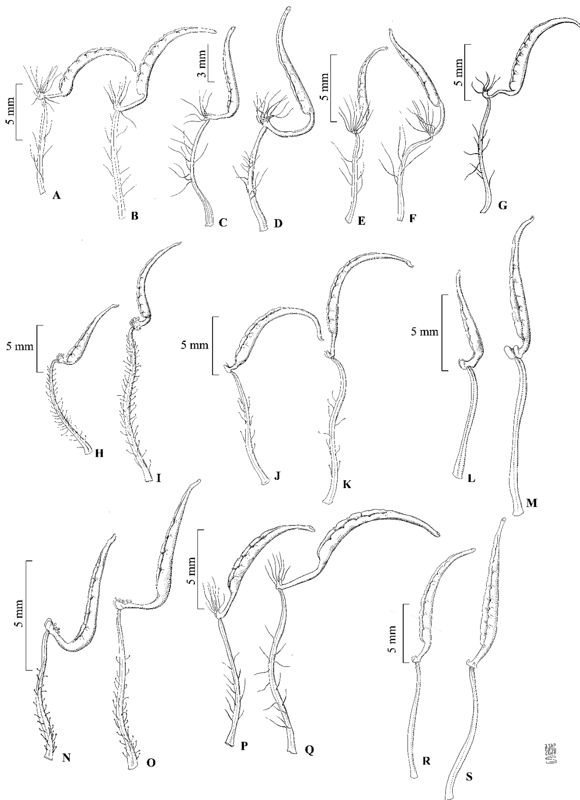
Figura 4. A-B: estame menor e maior de Tibouchina aegopogon ; C-D: estame menor e maior de T. albescens ; E-F: estame menor e maior de T. barbiger ; G: estame de T. bruniana ; H-I: estame menor e maior de T. candolleana ; J-K: estame menor e maior de T. crassiramis .
