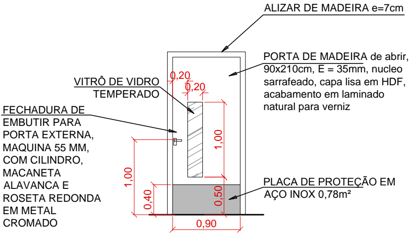
VISTA FRONTAL - P01 PORTAS DAS SALAS DE AULA NOVAS esc.: 1/50
