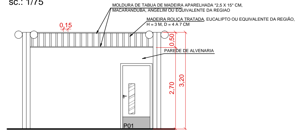
VISTA FRONTAL - VENEZIANAS DAS SALAS DE AULA sc.: 1/75
