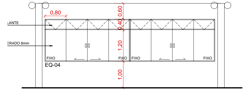
VISTA FRONTAL - EQ-04 sc.: 1/75
