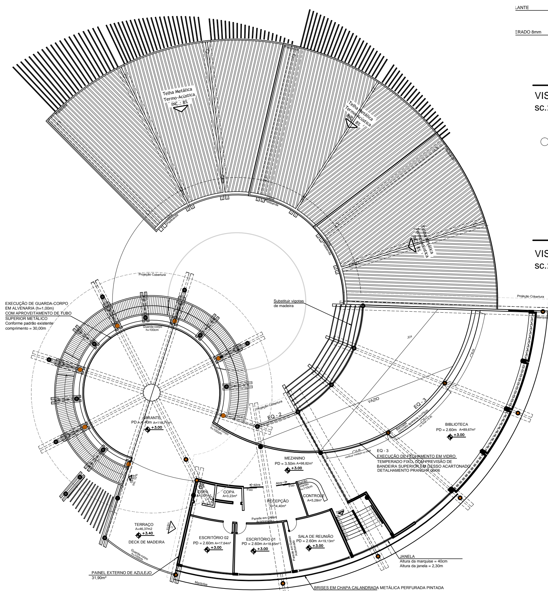
PLANTA BAIXA DO PAVIMENTO SUPERIOR esc.: 1/200
