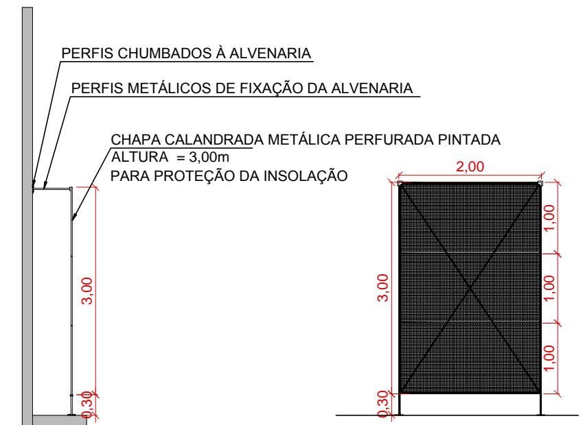
CORTE TRANSVERSAL CHAPA PERFURADA sc.: 1/75
