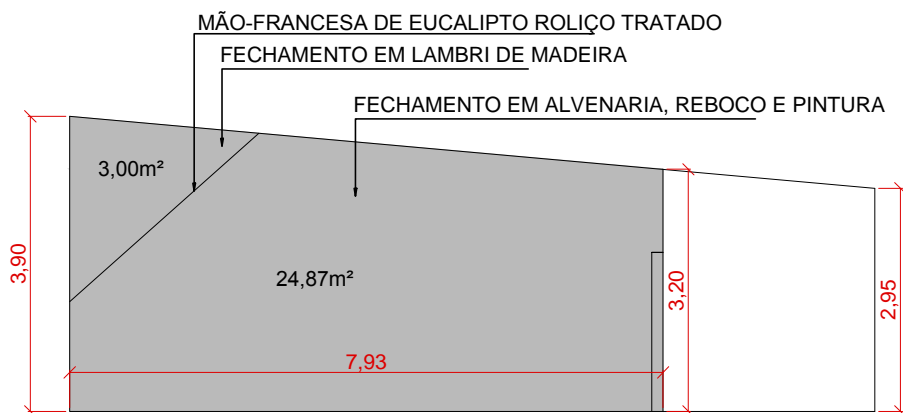
VISTA B - PAREDES INTERNAS DAS SALAS DE AULA TÉRREO esc.: 1/100
