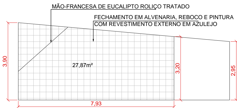
VISTA A - PAREDES EXTERNAS DAS SALAS DE AULA TÉRREO esc.: 1/100
