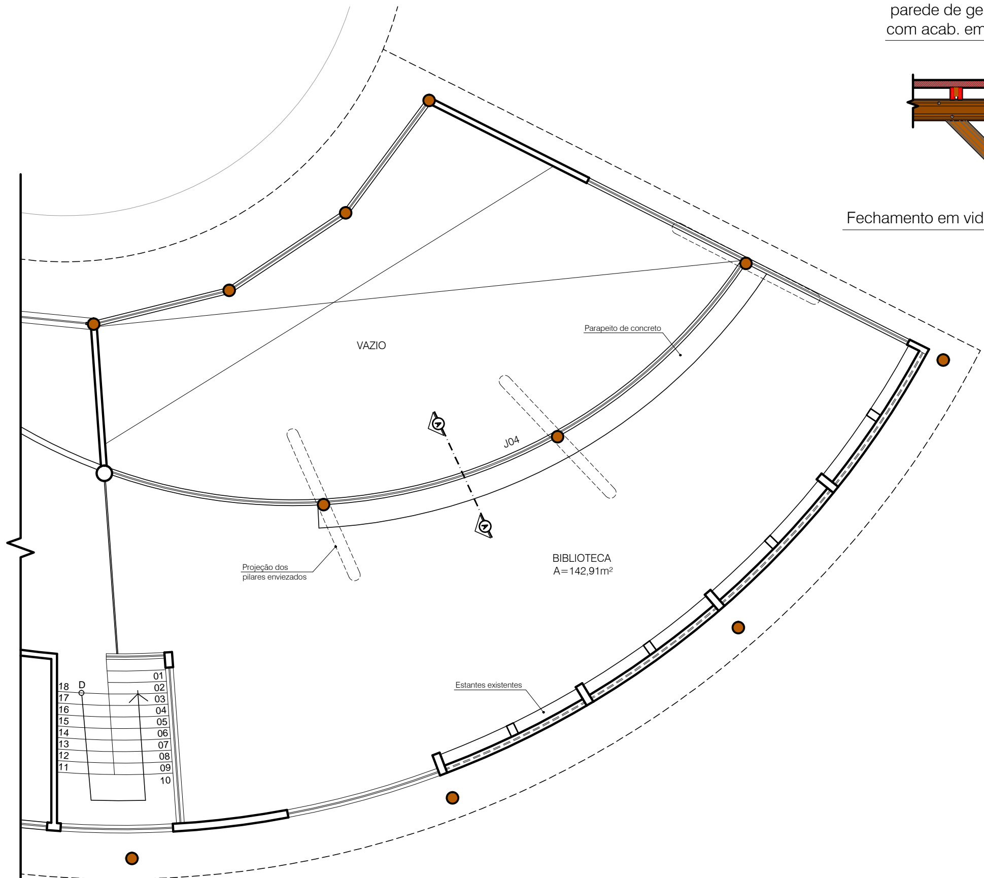
PLANTA BAIXA DO PAVIMENTO SUPERIOR esc.: 1/100
